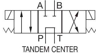
TANDEM CENTER
