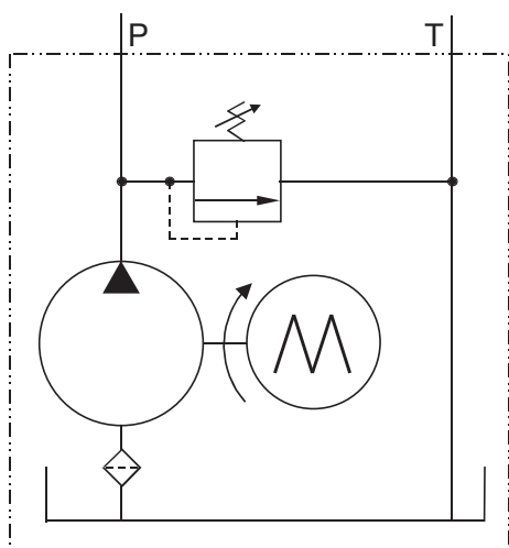
"SA" CIRCUIIT
